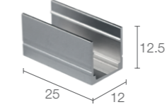
WTBAS002A Clip di fissaggio (1 pezzo) Mounting clip (1 piece)
