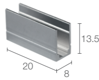
WTBAS000A Clip di fissaggio (1 pezzo) Mounting clip (1 piece)
