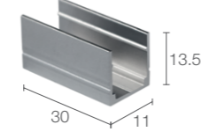
WTBAS001A Clip di fissaggio (1 pezzo) Mounting clip (1 piece)
