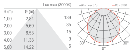
DD - Diffuse CRI 80
