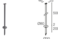
WP1006F Piquet pour installation au sol - h 500 mm - gris
