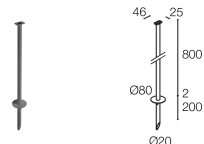
WP1007F Piquet pour installation au sol - h 800 mm - gris
