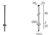
WP1007F Piquet pour installation au sol - h 800 mm - gris
