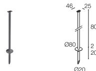
WP1007F Erdspeiß zur Bodenmontage - h 800 mm - grau
