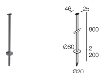
WP1007F Erdspeiß zur Bodenmontage - h 800 mm - grau
