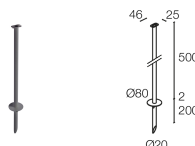
WP1006F Erdspeiß zur Bodenmontage - h 500 mm - grau
