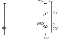
WP1006H Erdspeiß zur Bodenmontage - h 500 mm - anthrazit
