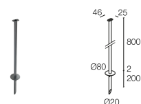
WP1007H Erdspeiß zur Bodenmontage - h 800 mm - anthrazit
