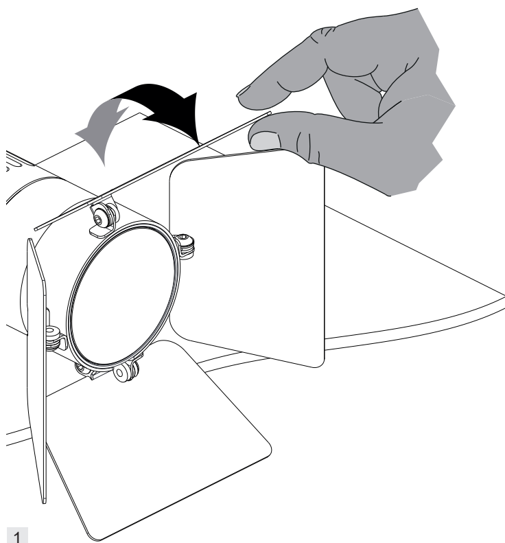
Tilt adjustment / Regolazione inclinazione / Réglage de l'inclinaison / Neigungsverstellung / Ajuste de la inclinación
