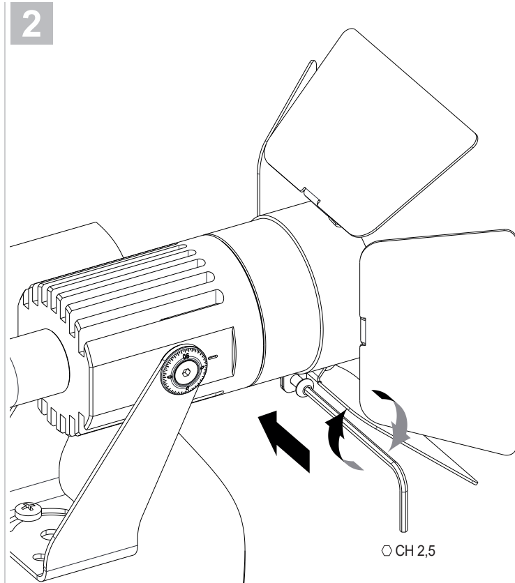
Tilt adjustment / Regolazione inclinazione / Réglage de l'inclinaison / Neigungsverstellung / Ajuste de la inclinación
